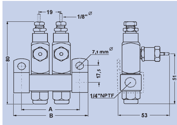
Размеры распределителя SL-32
