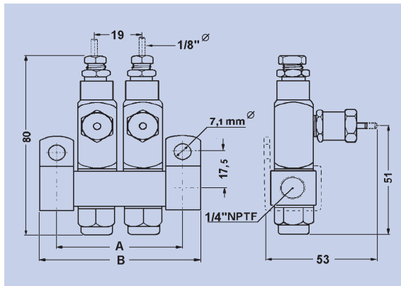
Размеры распределителя SL-43
